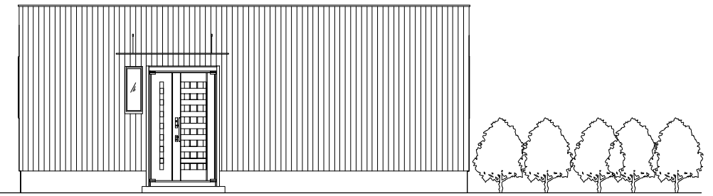
西側立面図 1 : 100
