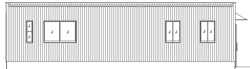
北側立面図 1 : 100
