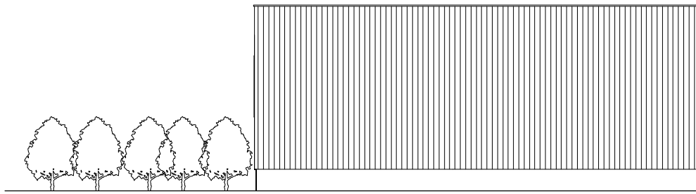
東側立面図 1 : 100
