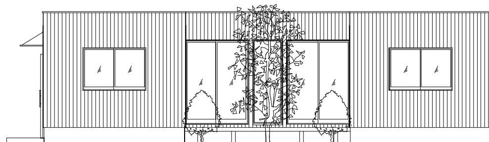
南側立面図 1 : 100
